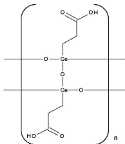
Figura 2. Dibujo esquemático mostrando la coordinación de los átomos de germanio en uno de los planos que constituyen la red del sesquióxido de carboxietilgermanio (Ge-132).
