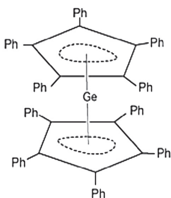
Figura 7. Estructura esquemática del decafenilgermanoceno.
