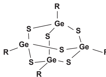
Figura 5. Estructura esquemática de los sesquisulfuros organogermánicos.
