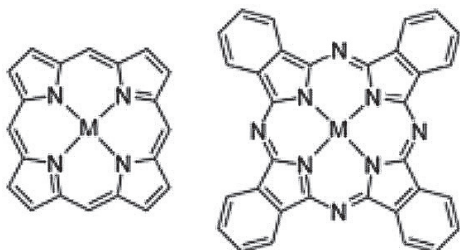
Figura 6. Complejos metálicos de la porfina (izq.) y de la ftalocianina (der.).
