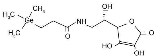
Figura 3. Estructura esquemática del compuesto denominado Ge-Vit.
