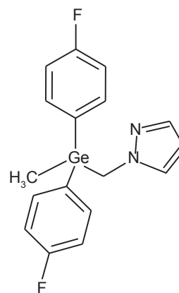
Figura 8. Estructura esquemática del germaflusilazol.
