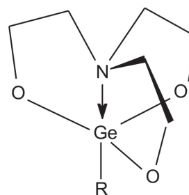
Figura 4. Estructura esquemática de los germatranos.
