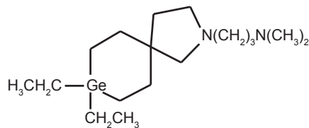
Figura 1. Estructura esquemática del spirogermanio.
