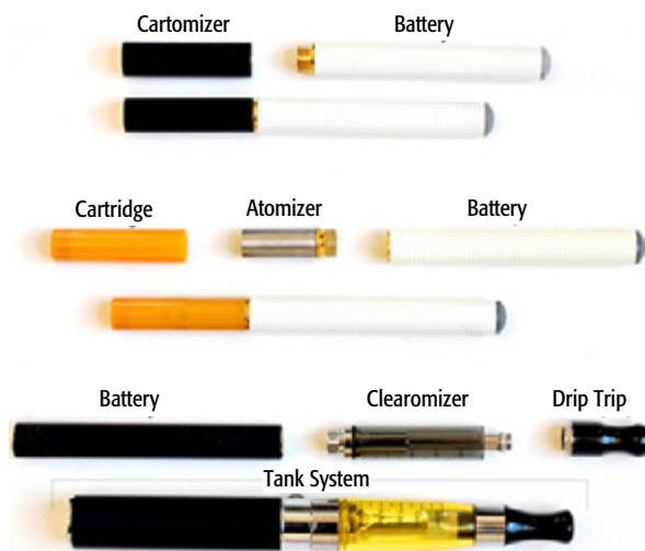
FIGURA 1. Cigarillo electrónico de primera generación.
